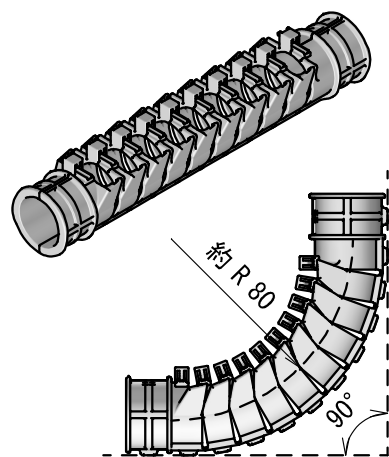
組立状態図
